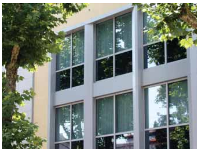
Facciata continua modello Ekonal con sistema di ante nascoste
